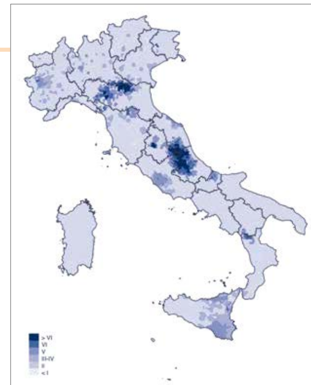
Principali terremoti che hanno colpito i Comuni italiani tra il 2008 e il 2022, classificati in base alla scala di intensità Mercalli.
